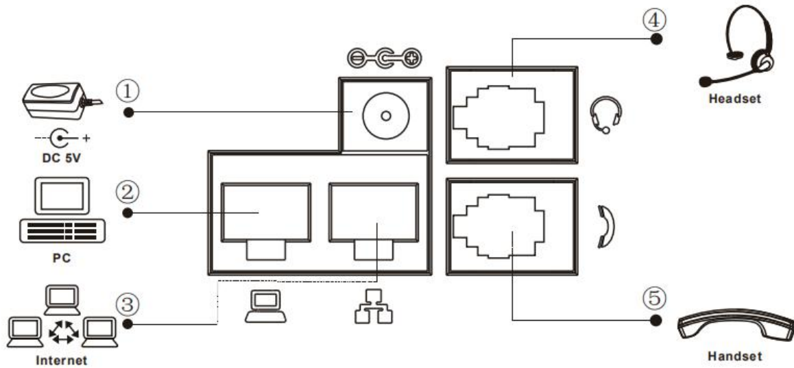
图 2 - 设备连接
